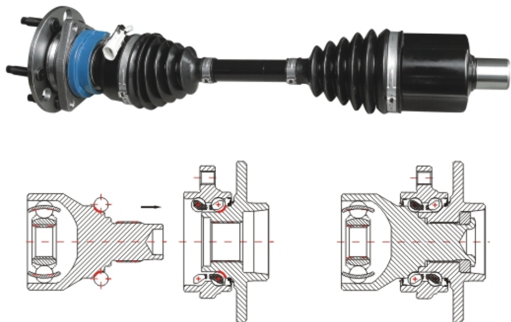
第四代汽车轮毂轴承单元（集成万向节） The 4 th generation hub assembly (with C.V. Joint)
